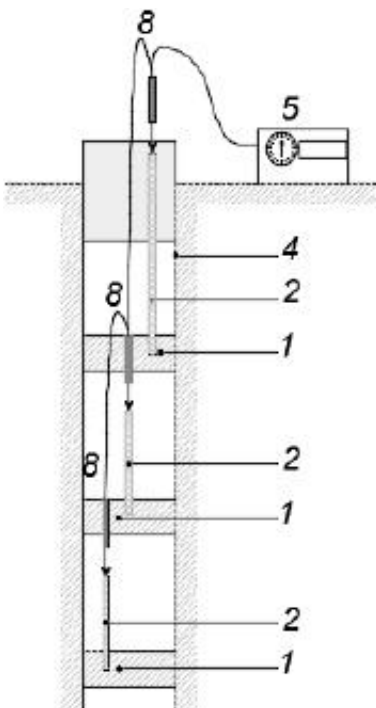
в) Звеньевой экстензометр
