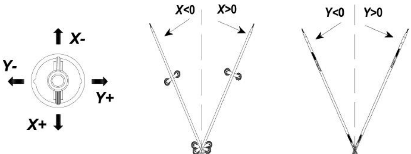
Рисунок Б.4 - Направления измерительных осей зонда скважинного инклинометра
