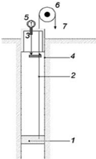
б) Проволочный экстензометр
