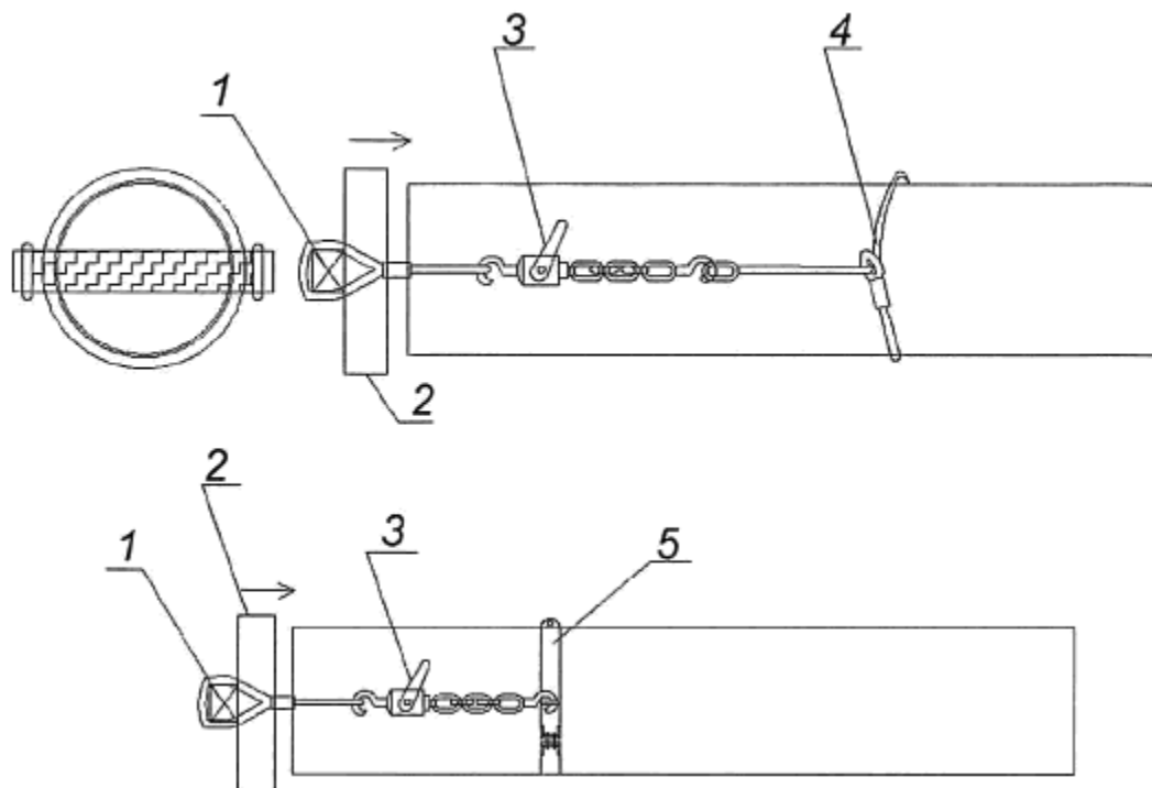
Рисунок 6 - Схема надевания муфты на трубу
